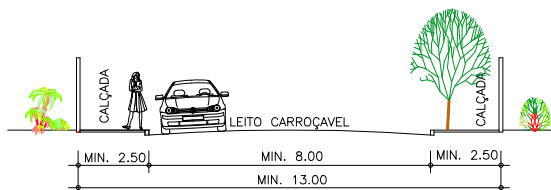
GABARITO ESPECIAL SEM ESCALA (VIAS LOCAIS EM EMPREENDIMENTOS DE INTERESSE SOCIAL)
