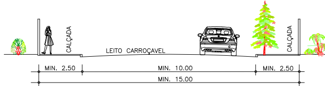
GABARITO 2 - PERFIL TRANSVERSAL - VIAS DE NO MÍNIMO DE 15,00 METROS SEM ESCALA
