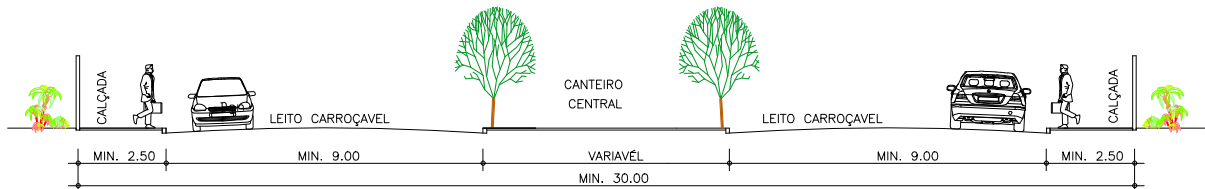
GABARITO 4 - PERFIL TRANSVERSAL - VIAS DE NO MÍNIMO DE 30,00 METROS SEM ESCALA
