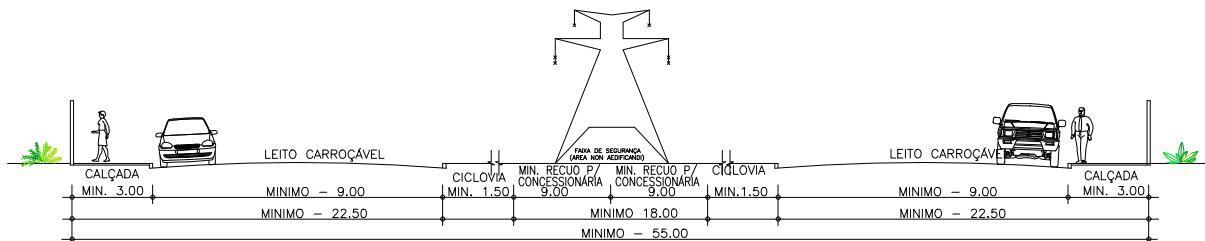
GABARITO 6 - FAIXA DE SERVIÇÃO ALTA TENSÃO (A SER DEFINIDO PELA CONCESSIONÁRIA) SEM ESCALA
