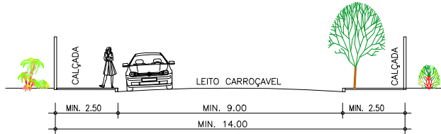
GABARITO 1 - PERFIL TRANSVERSAL - VIAS DE NO MÍNIMO DE 14,00 METROS SEM ESCALA
