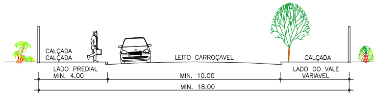
GABARITO 3 - PERFIL TRANSVERSAL - VIAS DE NO MÍNIMO DE 18,00 METROS SEM ESCALA
