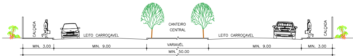
GABARITO 5 - PERFIL TRANSVERSAL - VIAS DE NO MÍNIMO DE 50,00 METROS SEM ESCALA
